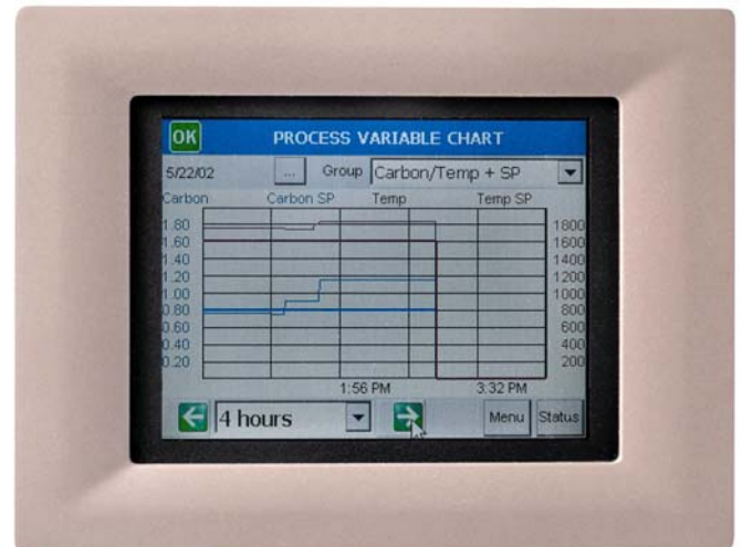
Tela Gráfica Típica
